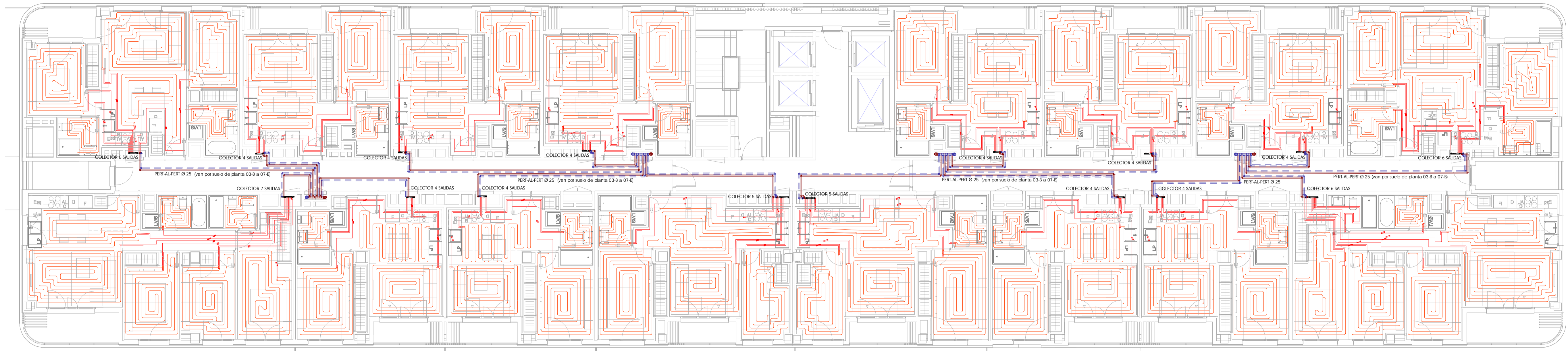
2 PLANTA TIPO BLOQUE B. 03-B-04-B-05-B-06-B Y 07-B 1:100
