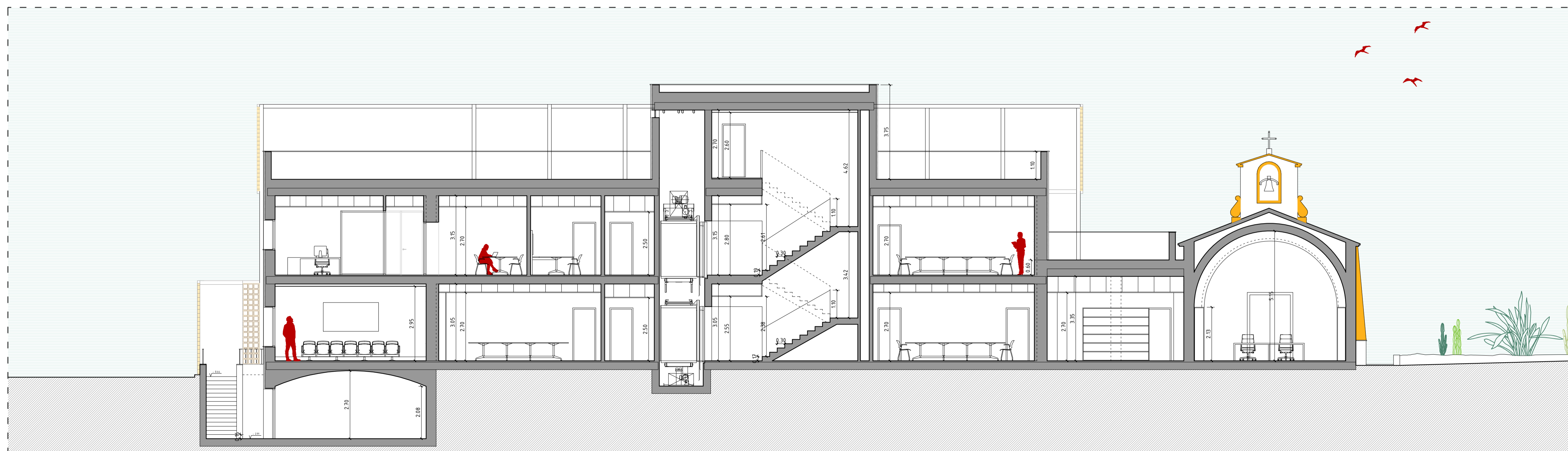
SECCIÓN 1
